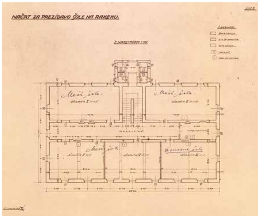
Načrt za prezidavo šole na Rakeku, I. nadstropje, junij 1928, hrani Slovenski šolski muzej (SSM).
